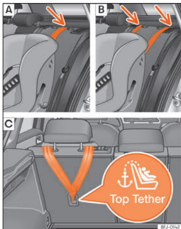
Fig. 28 Yderste siddepladser på 2. sæderække: indstilling og monteringsafhængigt af Top Tether-rem
