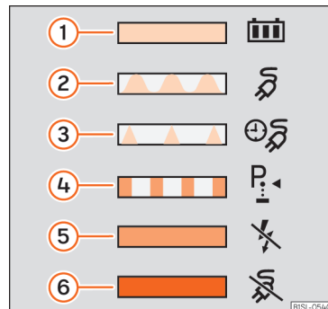
Fig. 229 På indersiden af batteriladeklappen: mærkat med informationer vedr. opladningsindikatoren
