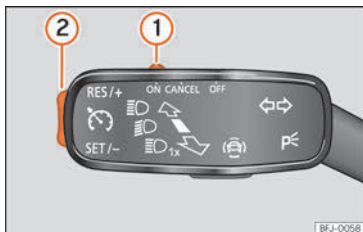
Fig. 179 På blinklysarmen: betjeningselementer til betjening af fartpiloten
