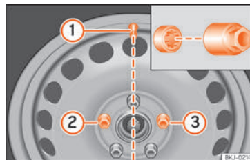
Fig. 36 Hjulskift: dækventil ① og placering af låsebolt ② eller ③
