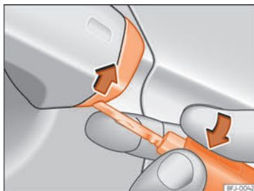
Fig. 80 Førerdørens dørhåndtag: Sådan vipes afdækningen af.
