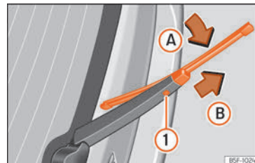
Fig. 42 Udskiftning af viskerblad til bagrude
