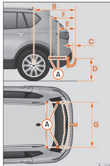
Fig. 221 Mål og fastgørelsespunkter for eftermontering af anhængertræk
