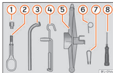
Fig. 31 I bagagerummet under bagagerumbunden: bilens værktøj
