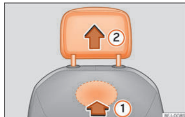
Fig. 108 Hovedstøtter foran: afmontering
