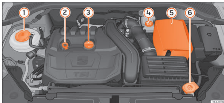
Fig. 240 Elementernes placering
