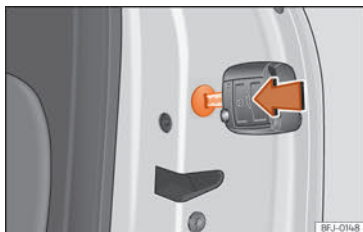
Fig. 81 Dørnødlås
