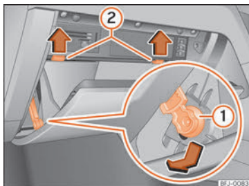
Fig. 50 Handskerum (højrestyret bil): adgang til sikringsboksen
