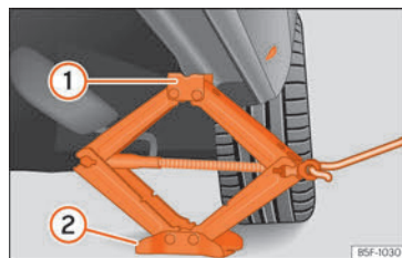
Fig. 38 Længdevange: påsætning af donkraft
