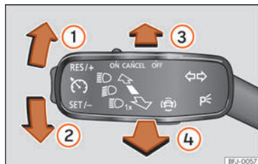
Fig. 94 Blink- og fjernlysarm
