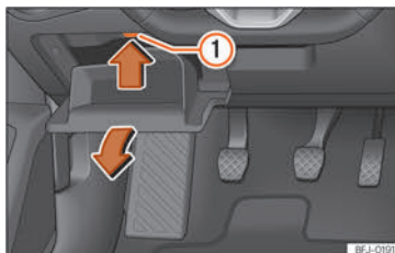
Fig. 49 Instrumentpanelet i førersiden (venstrestyret bil): afdækning på sikringsboks
