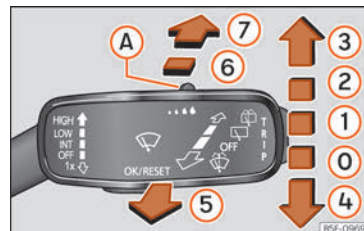
Fig. 97 Betjening af forrude- og bagrudeviskere
