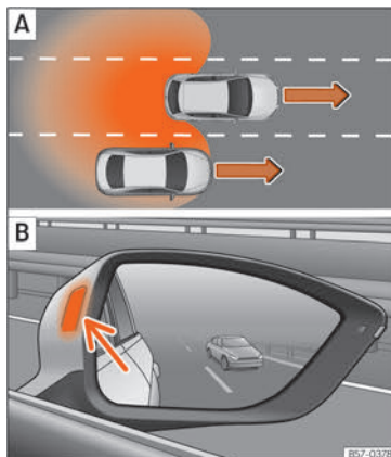
Fig. 197 Skematisk visning: A Overhaling og efterfølgende skift til højre vognbane. B Indikator til vognbaneskiftassistenten i højre sidespejl
