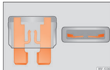
Fig. 52 Sikring, der er brændt over
