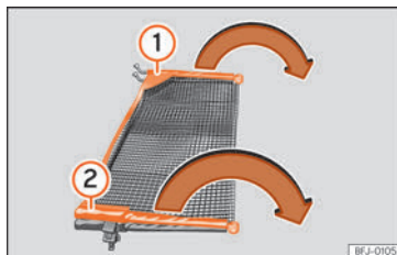
Fig. 130 Udklapning af netskillevæg
