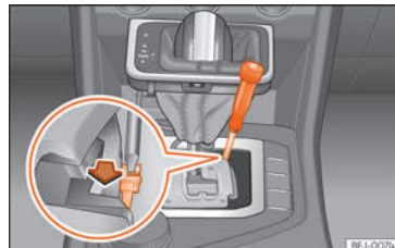
Fig.169 Gearvælger: nødoplåsning fra parkeringsposition
