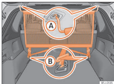
Fig. 132 Monteret netskillevæg
