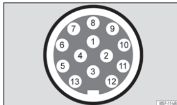
Fig. 219 Skematisk visning: tilhørsforhold for stikben i anhængerstikdåsen
