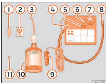
Fig. 32 Principskitse: havarisættets dele
