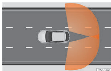
Fig. 176 Sensorernes registreringsområde
