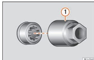
Billede 196 Låsebolt med dækkappe og adapter
