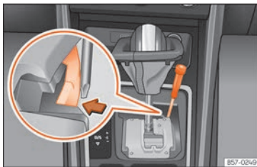
Billede 90 Gearvælger: nødoplåsning fra parkeringsposition
