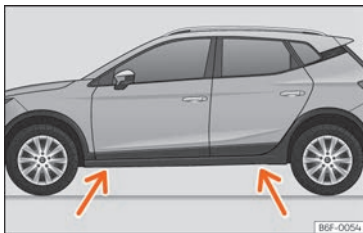
Billede 199 Løftepunkter til donkraften.
