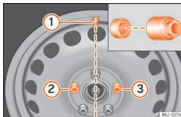
Billede 198 Hjulskit: dækventil ① og placering for låsebolt ② eller ③
