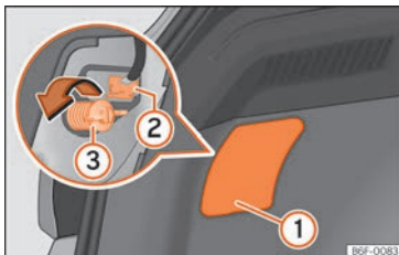
Billede 172 Bagagerum: adgang til skrue til baglygte
