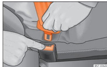
Billede 24 Frigørelse af låsetap fra selelåsen
