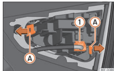
Billede 175 Afmontering af pæreholder
