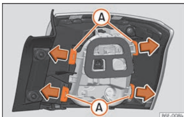
Billede 173 Fastgørelsestapper på bagsiden af baglygten
