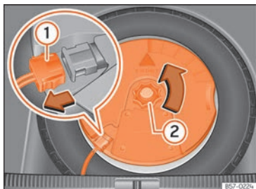
Billede 193 I bagagerummet: afmontering af subwoofer
