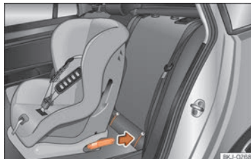
Billede 38 Bagsæde: montering af børnesæde med ISOFIX-system
