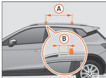
Billede 150 Fastgørelsespunkter til længdevangerne til tagbøjlesystemet
