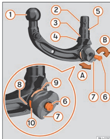
Billede 156 Oversigt: aftageligt anhængertræk
