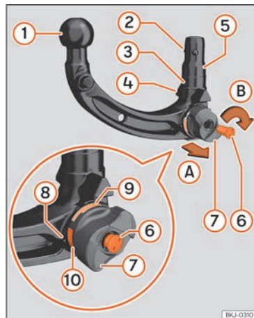
Billede 155 Oversigt: aftageligt anhængertræk
