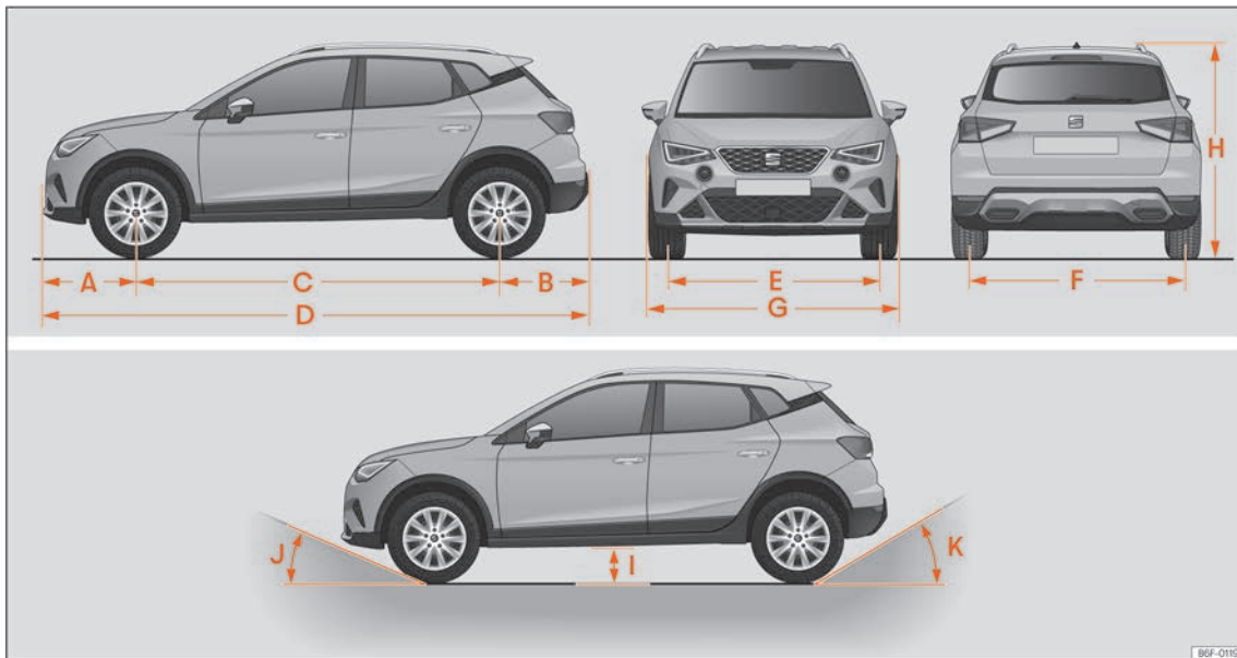
Billede 206 Mål og vinkler
