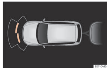
Billede 121 Parkeringshjælpens skærmvisning ved kørsel med anhænger.
