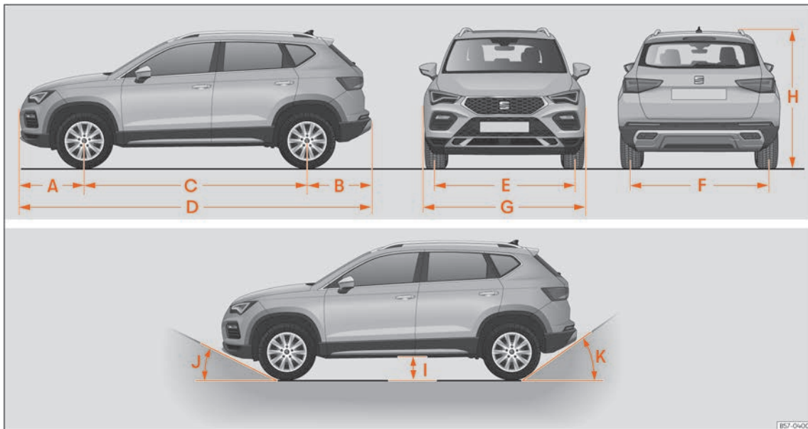
Billede 235 Mål
