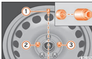
Billede 227 Hjulskift: dækventil ① og placering for låsebolt ② eller ③
