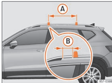
Billede 182 Fastgørelsespunkter til længdevangerne til tagbøjlesystemet
