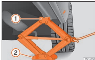
Billede 229 Længdevange: påsætning af donkraft
