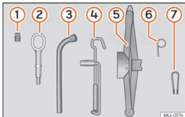
Billede 191 I bagagerummet under bagagerumsbunden: bilens værktøj
