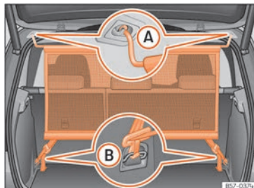
Billede 175 Monteret netskillevæg
