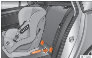
Billede 40 Bagsæde: montering af børnesæde med ISOFIX-system
