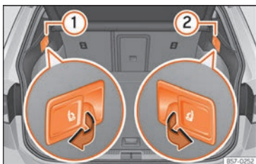
Billede 81 | bagagerummet: greb til udløsning af bagsæderyglæn
