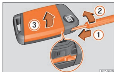
Billede 49 Bilnøgle: åbning af afdækning til batterium
