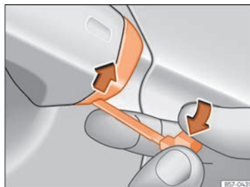
Billede 56 Førerdørens dørhåndtag: Sådan vippes afdækningen af.
