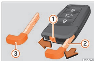
Billede 48 Bilnøgle: udtagning af nødnøgle
