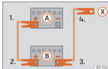
Billede 195 Tilslutningsdiagram for biler uden start-stop-system
