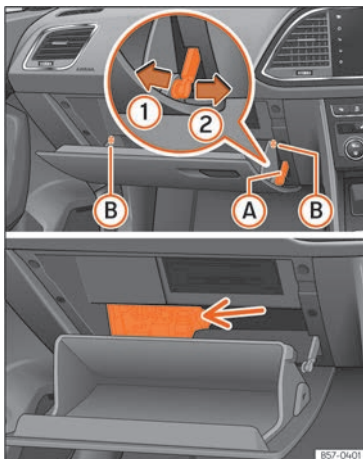
Billede 202 Højrestyret bil: afdækning til sikringsboks i instrumentpanelet i passagersiden
