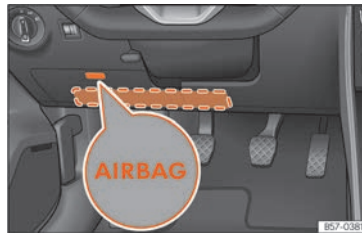
Billede 34 | I førersiden: knæairbaggens monteringssted
