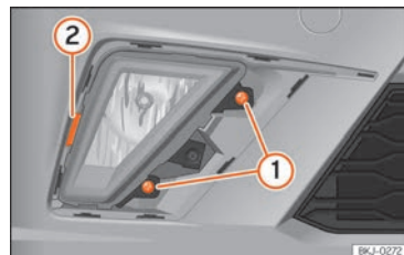
Billede 167 Tågeforlygte: afmontering af pæreholder
