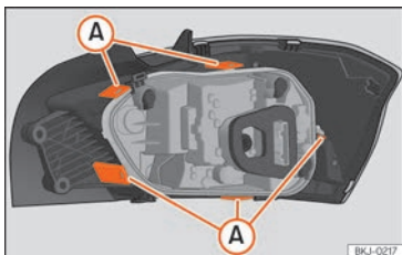
Billede 165 Fastgørelsestapper på bagsiden af baglygten
