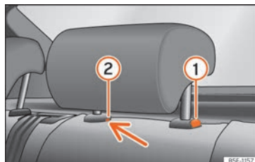
Billede 70 Hovedstøtte bag: afmontering
