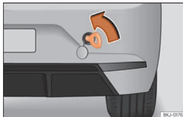
Billede 160 I højre side af den bageste stødfanger: slæbeøje, der er skruet i
