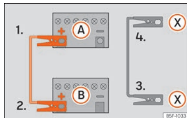
Billede 156 Tilslutningsdiagram for biler med start-stop-system
