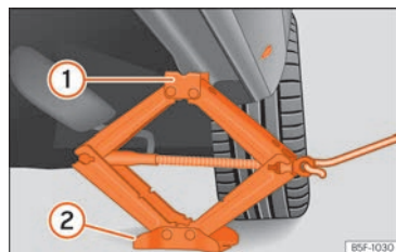
Billede 193 Længdevange: påsætning af donkraft
