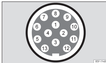
Billede 145 Skematisk visning: tilhørsforhold for stikben i anhængerstikdåsen
