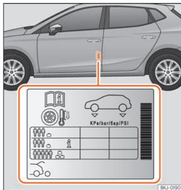
Billede 182 Placering af mærkatene med dæktryk.
