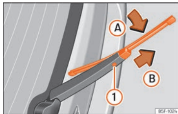
Billede 154 Udskiftning af viskerblad til bagrude
