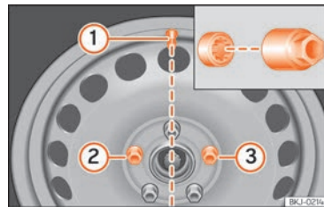
Billede 191 Hjulsift: dækventil ① og placering for låsebolt ② eller ③
