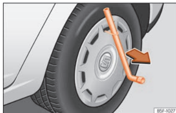
Billede 187 Tag hjulkapslen af hjulet.
