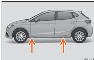
Billede 192 Løftepunkter til donkraften.
