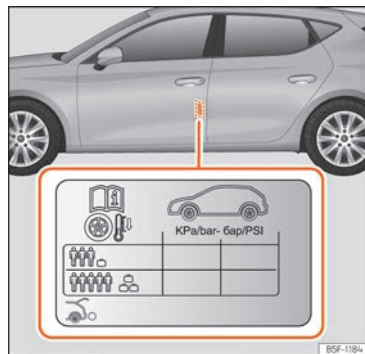
Billede 238 Placering af mærkaten med dæktryk.
