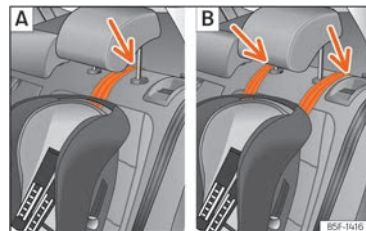
Billede 48 Bagsædepladser: indstilling og montering ved anvendelse af Top Tether-rem
