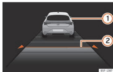
Billede 135 På kombiinstrumentets skærm: ACC aktiv
