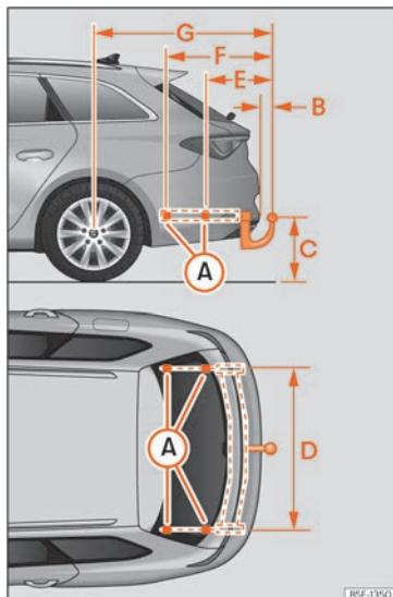
Billede 207 Mål og fastgørelsespunkter for eftermontering af anhængertræk
