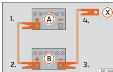
Billede 215 Tilslutningsdiagram for biler uden start-stop-system
