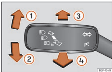
Billede 105 Blink- og fjernlysarm
