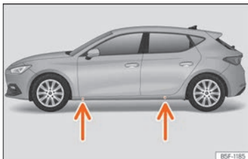
Billede 248 Løftepunkter til donkraften.
