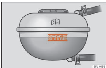
Billede 227 I fronttrummet: markeringer på kølevæskeekspansionsbeholderen
