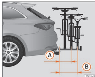
Billede 206 Skematisk visning af maksimalt udhæng for lasten på en cykelholder til to eller tre cykler.
