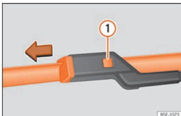
Billede 214 Udskiftning af viskerblade foran
