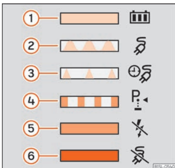
Billede 63 På indersiden af batteriladeklappen: mærkat med informationer vedr. opladningsindikatoren
