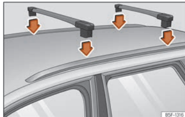
Billede 201 Fastgørelsespunkter til tagrælinger til tagbøjlesystemet (Leon Sportstourer)
