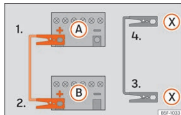
Billede 216 Tilslutningsdiagram for biler med start-stop-system
