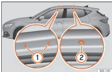
Billede 202 Fastgørelsespunkter i tagræling til tagbøjlesystemet (Leon)
