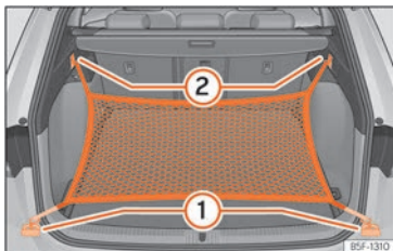
Billede 196 I bagagerummet: øjer ① og kroge ② til fastgørelse af bagagenet
