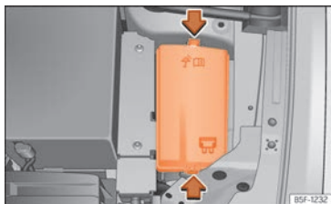
Billede 222 I motorrummet: afdækning på sikringsboks
