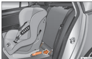
Billede 45 Bagsæde: montering af børnesæde med ISOFIX-system
