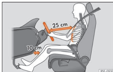
Billede 19 Der skal være en afstand på mindst 25 cm (10 inches) mellem føreren og rattet.
