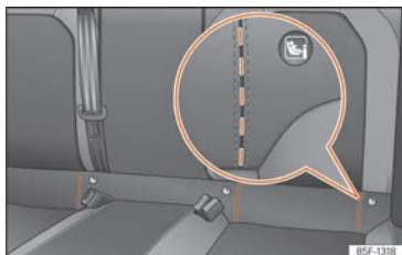
Billede 43 Bagsæde: præget slidspor til adgang til ISOFIX/i-Size-holdeøj
