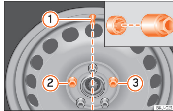
Billede 196 Hjulskift: dækkventil ① og placering for låsebolt ② eller ③
