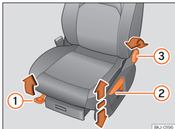
Billede 64 Forsæder: manuel sædeindstilling
