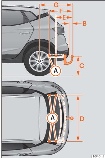
Billede 151 Mål og fastgørelsespunkter for eftermontering af anhængertræk
