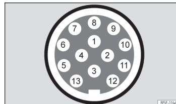
Billede 148 Skematisk visning: tilhørsforhold for stikben i anhængerstikkåsen
