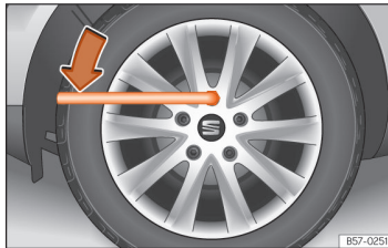
Billede 195 Hjulskift: løsning af hjulbolte
