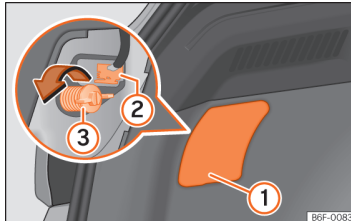
Billede 170 Bagagerum: adgang til skrue til baglygte
