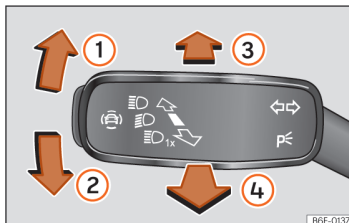
Billede 72 Blink- og fjernlysarm
