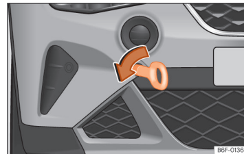
Billede 164 | Højre side af den forreste stødfanger: slæbeøj, der er skruet i
