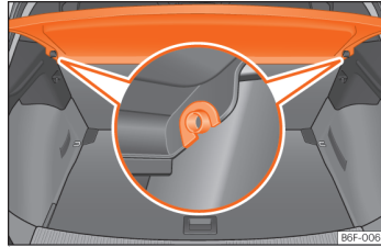
Billede 143 I bagagerummet: af- og påmontering af bagagerumsafdækning
