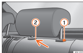
Billede 69 Hovedstøtte bagi: afmontering
