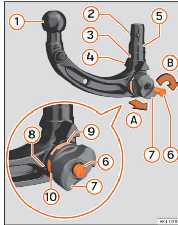
Billede 153 Oversigt: aftageligt anhængertræk
