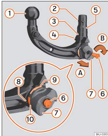
Billede 152 Oversigt: aftageligt anhængertræk
