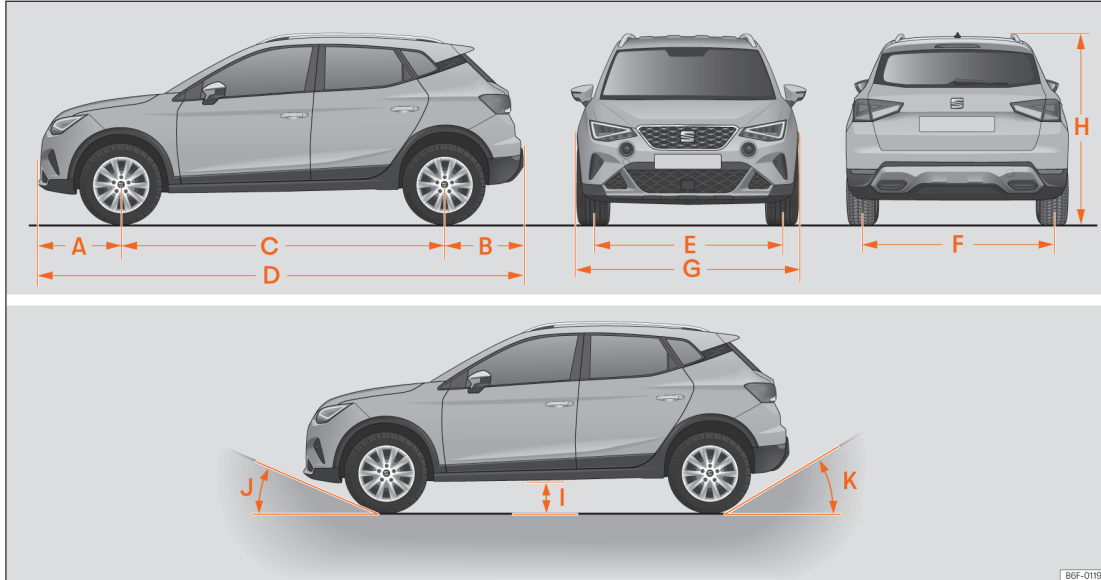
Billede 201 Mål og vinkler
