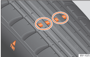
Billede 189 Dækprofil: slidindikatorer
