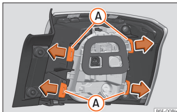
Billede 171 Fastgørelsestapper på bagsiden af baglygten
