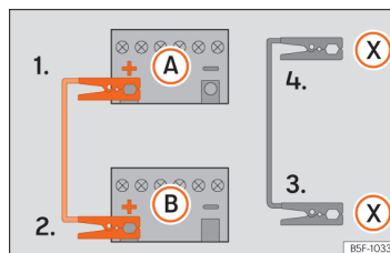
Billede 162 Tilslutningsdiagram for biler med start-stop-system
