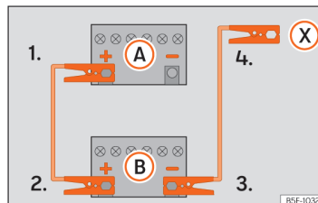
Billede 161 Tilslutningsdiagram for biler uden start-stop-system
