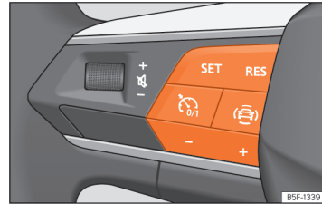
Billede 101 På multifunktionsrattet: knapper til betjening af hastighedsbegrænsere
