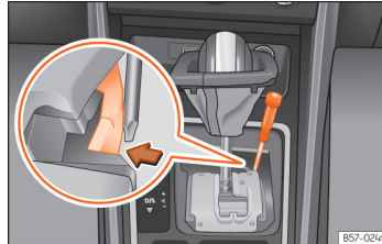
Billede 90 Gearvælger: nødoplåsning fra parkeringsposition
