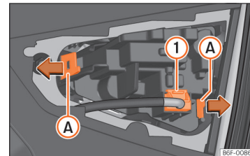
Billede 173 Afmontering af pæreholder
