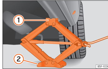
Billede 198 Længdevange: påsætning af donkraft
