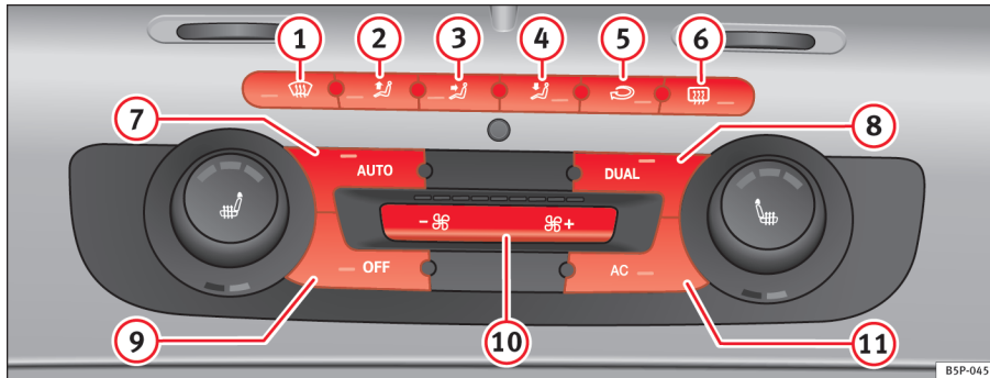
Fig. 130 I instrumentpanelet: betjeningslementer til 2C-Climatronic
