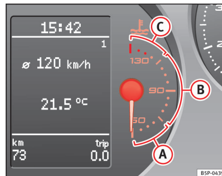
Fig. 35 Kombiinstrument: kølevæsketermometer
