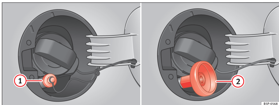
Fig. 158 Åbnet tankklap med påfyldningsstuds til autogas og adapter
