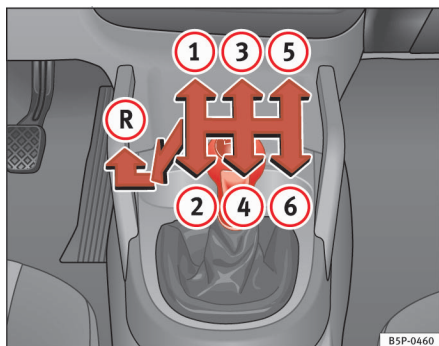
Fig. 142 I midterkonsollen: gearskiftediagram for en 6-trins manuel gearkasse
