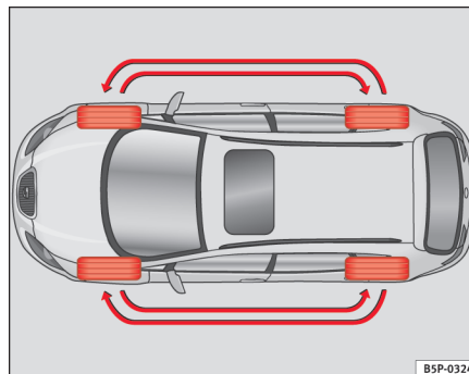
Fig. 174 Skema for ombytning af hjul
