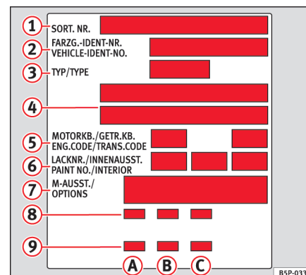
Fig. 207 Bilens datamærkat – bagagerum
