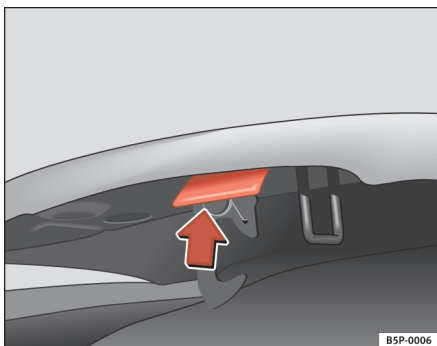
Fig. 162 Arm til motorhjelmen
