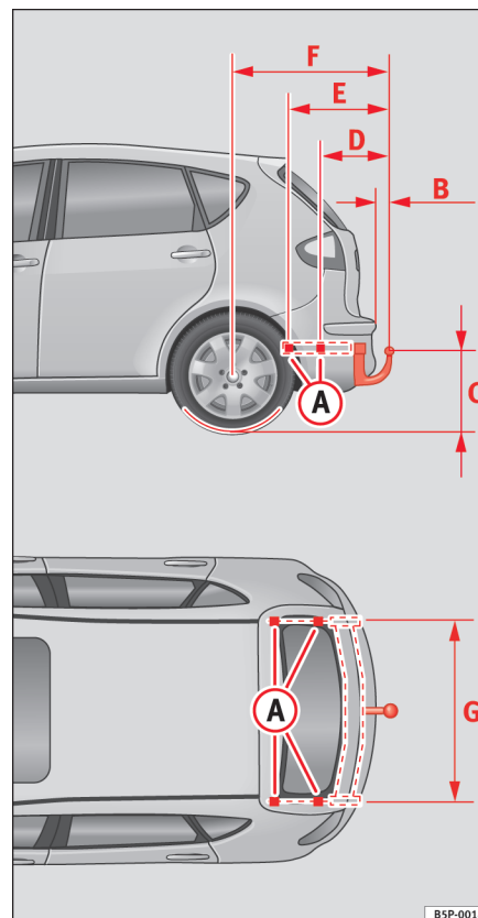
Fig. 156 Anhængertræk- kets fastgørelsespunkter ►
