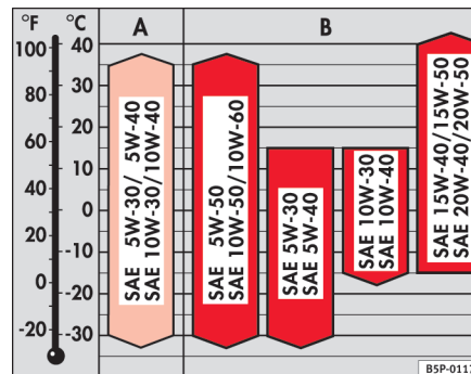
Fig. 163 Olietyper fordelt på temperaturområder
