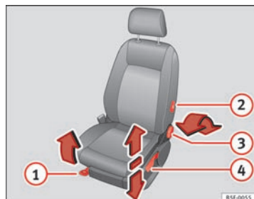
Fig. 71 Forsæder: manuel sædeindstilling
